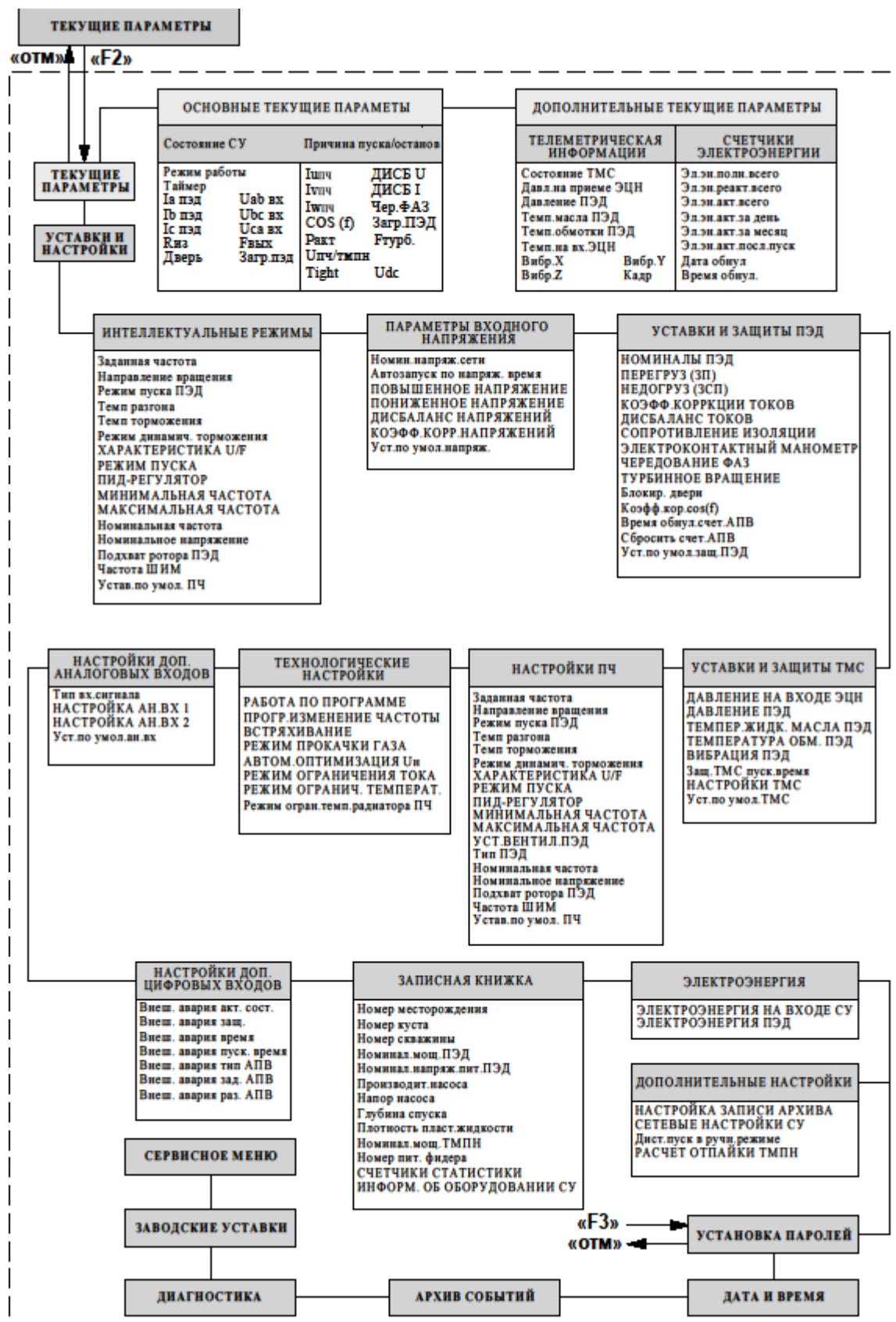
Рисунок А.1 – Структура меню СУ ИР3-540
