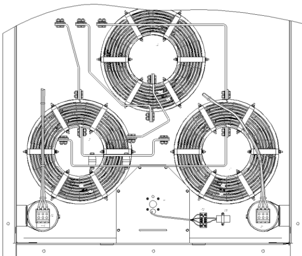
Рисунок Д.3 – СУ ИРЗ-545-02
