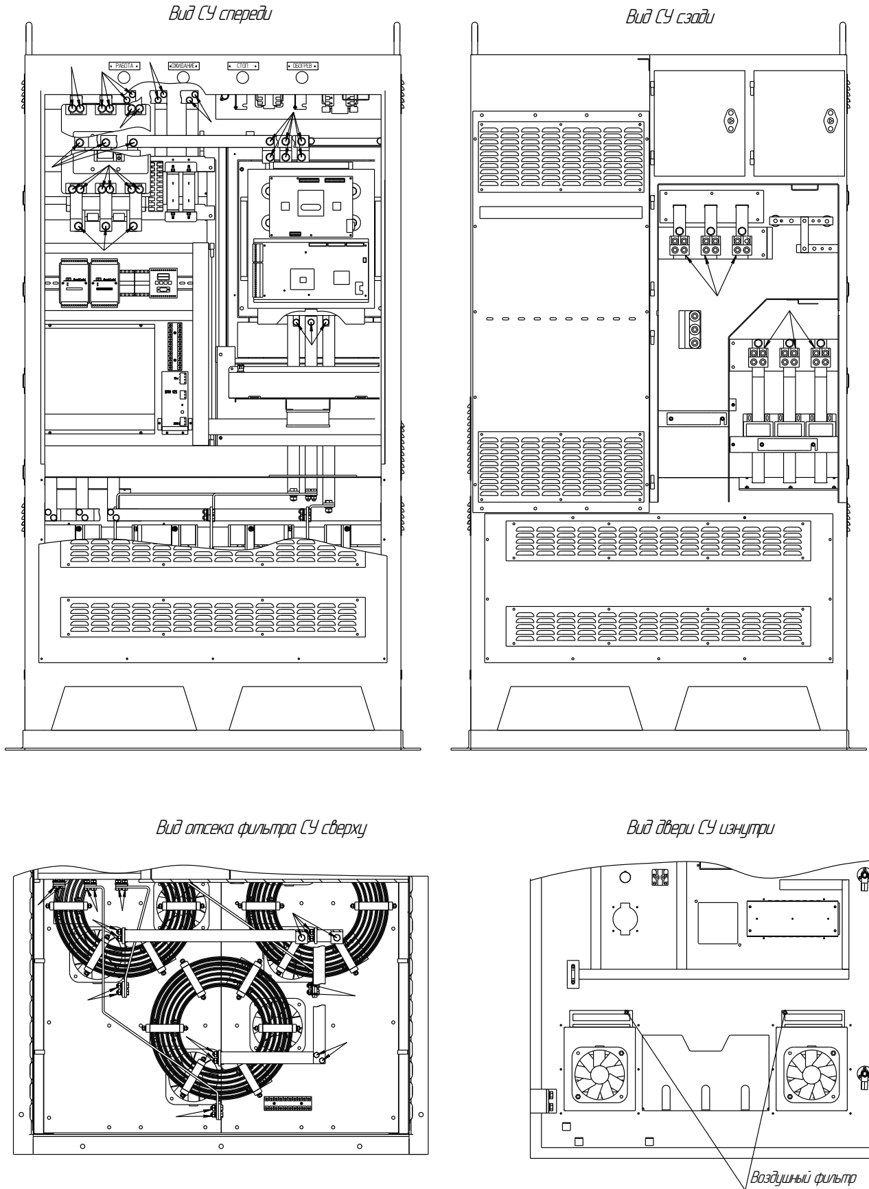
Рисунок Д.2 – СУ ИРЗ-541-02, ИРЗ-542-02
