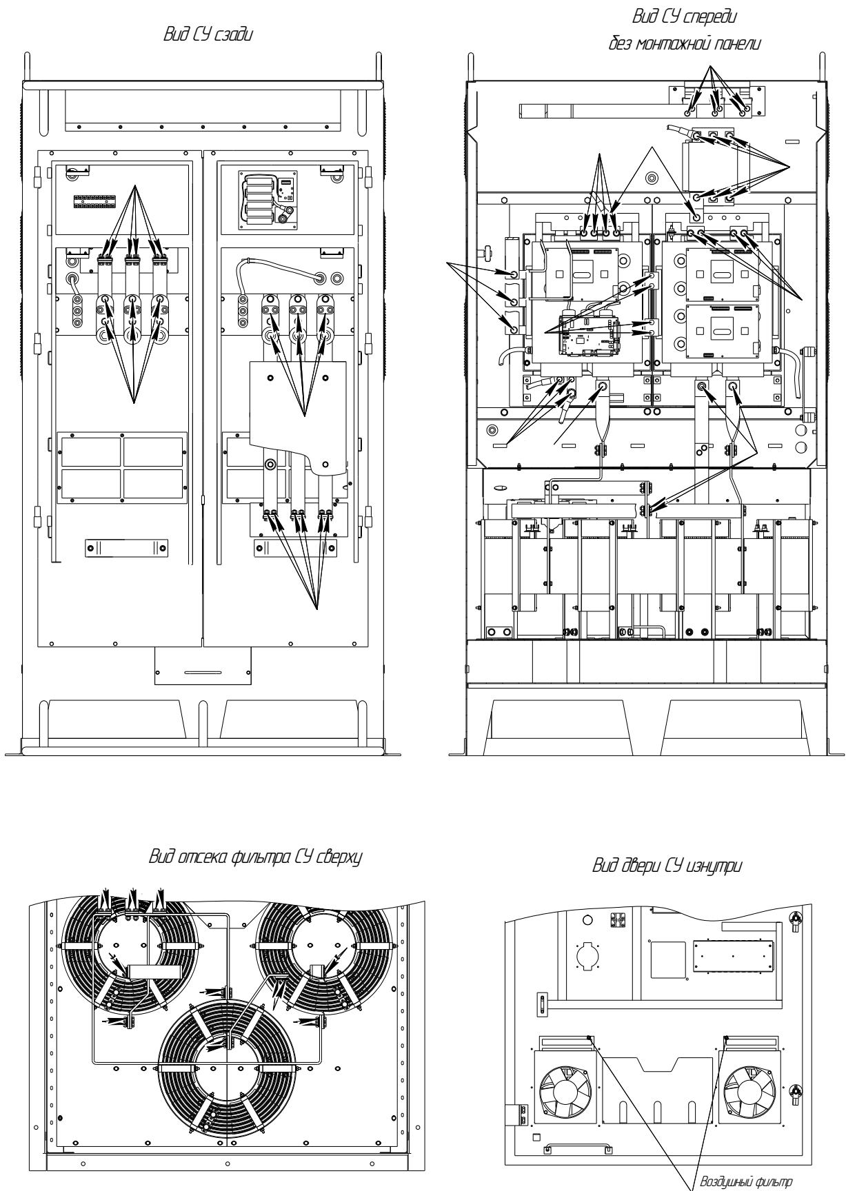
Рисунок Д.1 – СУ ИРЗ-543-02, ИРЗ-544-02
