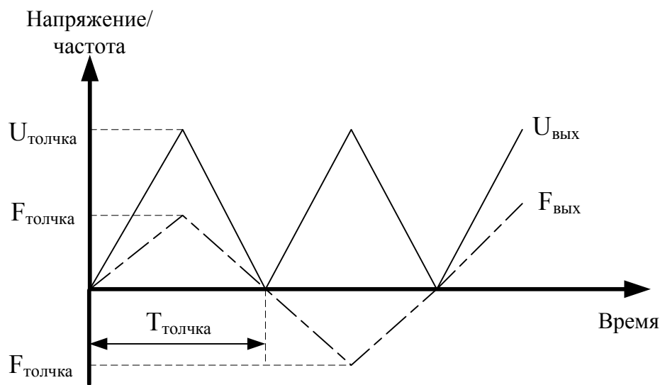
Рис. 2.2 Запуск ПЭД в режиме раскачки
