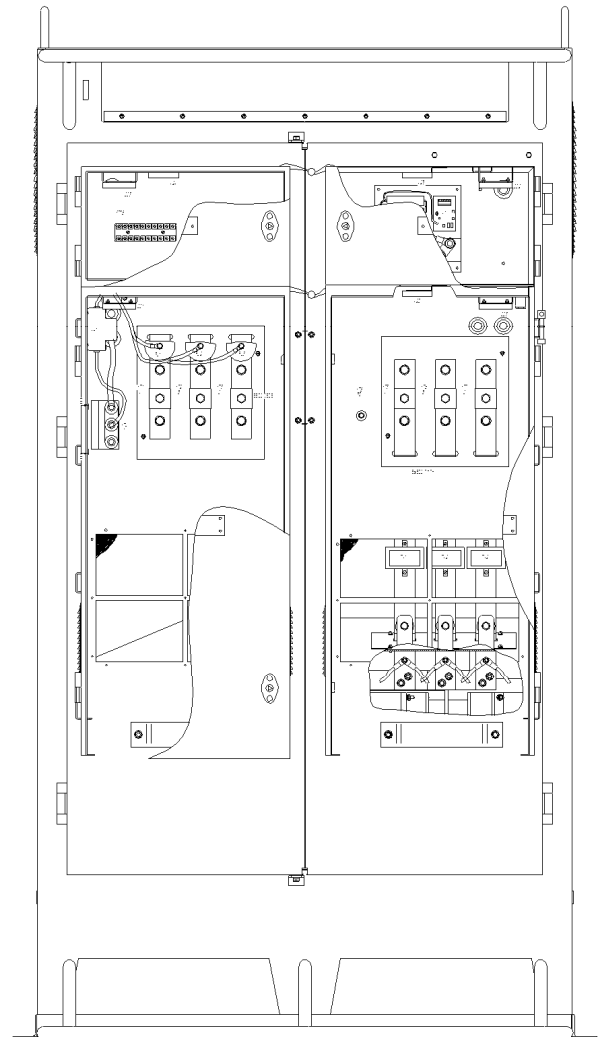
Вид СУ сзади
