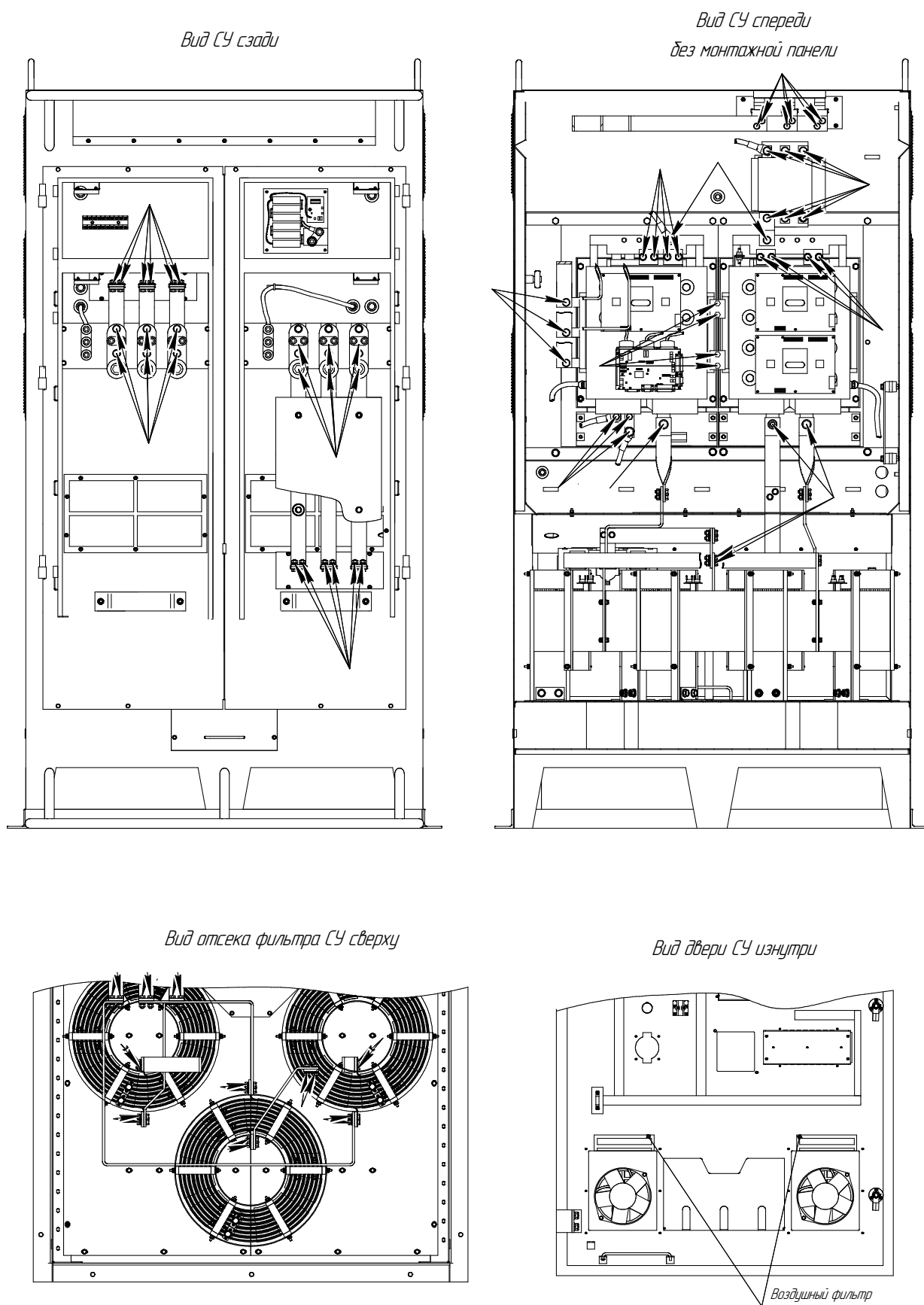
Рисунок Д.1 – СУ ИРЗ-553, ИРЗ-554
