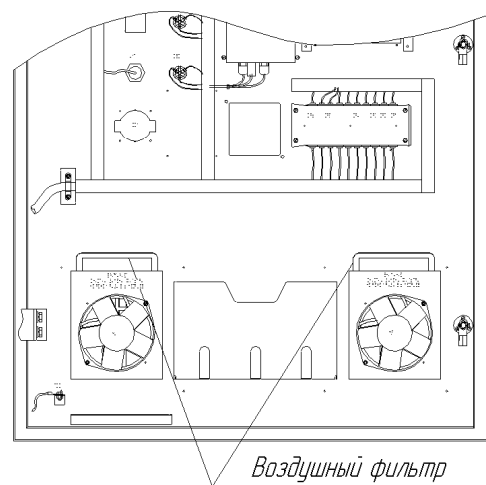
Вид двери СУ изнутри
