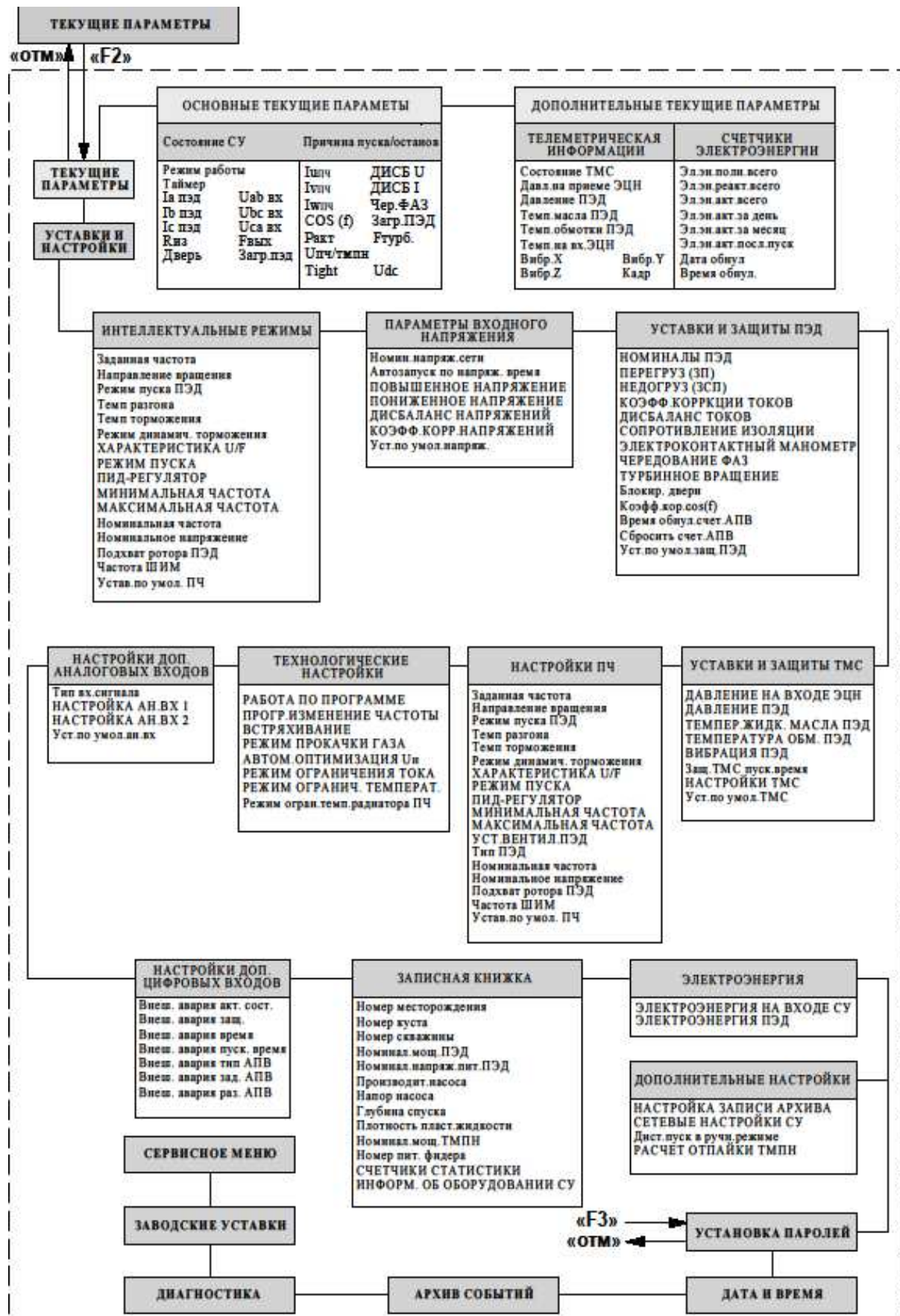
Рисунок А.1 – Структура меню СУ ИР3-550
