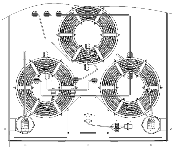
Вид отсека фильтра СУ сверху
