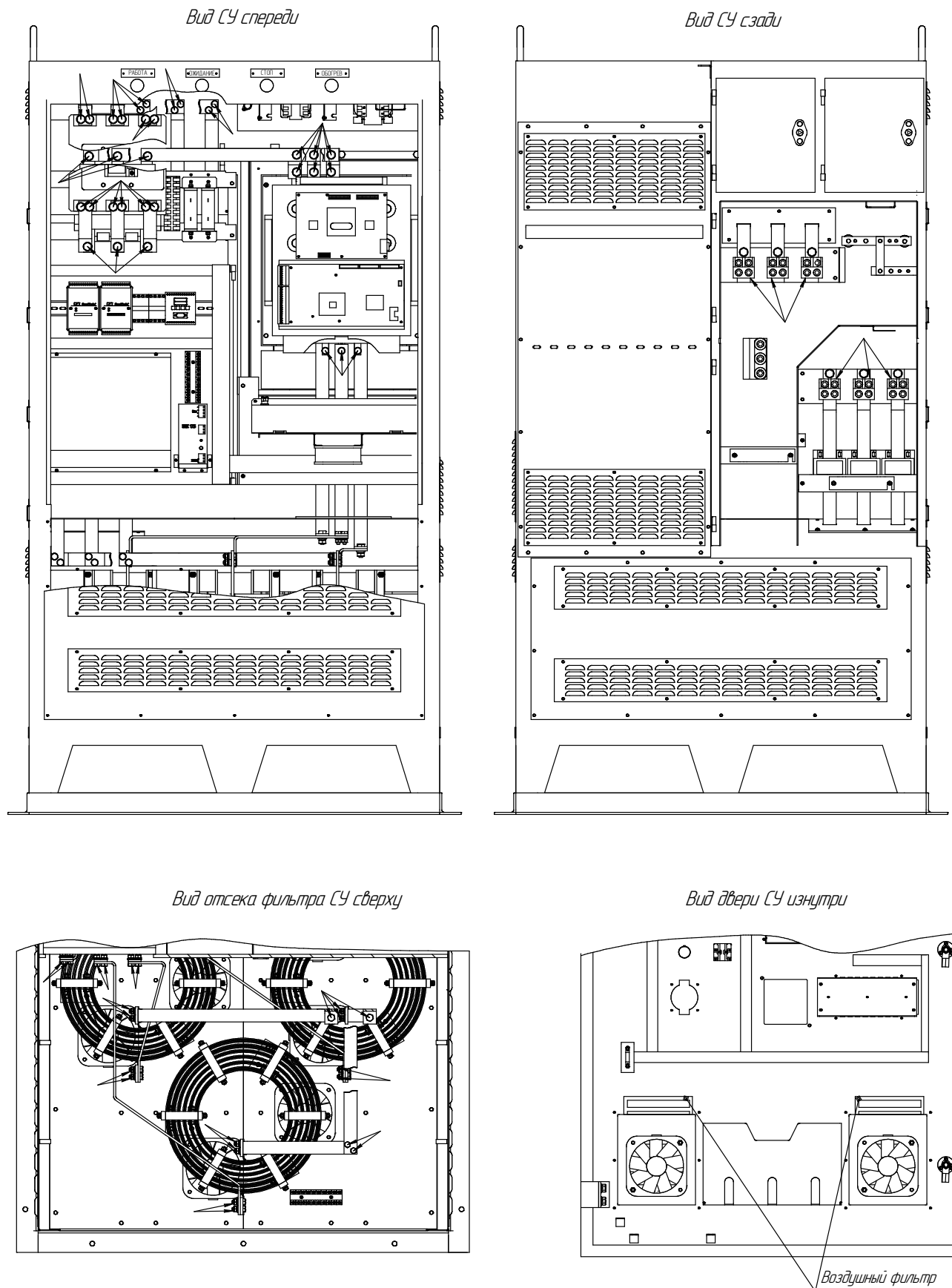
Рисунок Д.2 – СУ ИРЗ-551, ИРЗ-552
