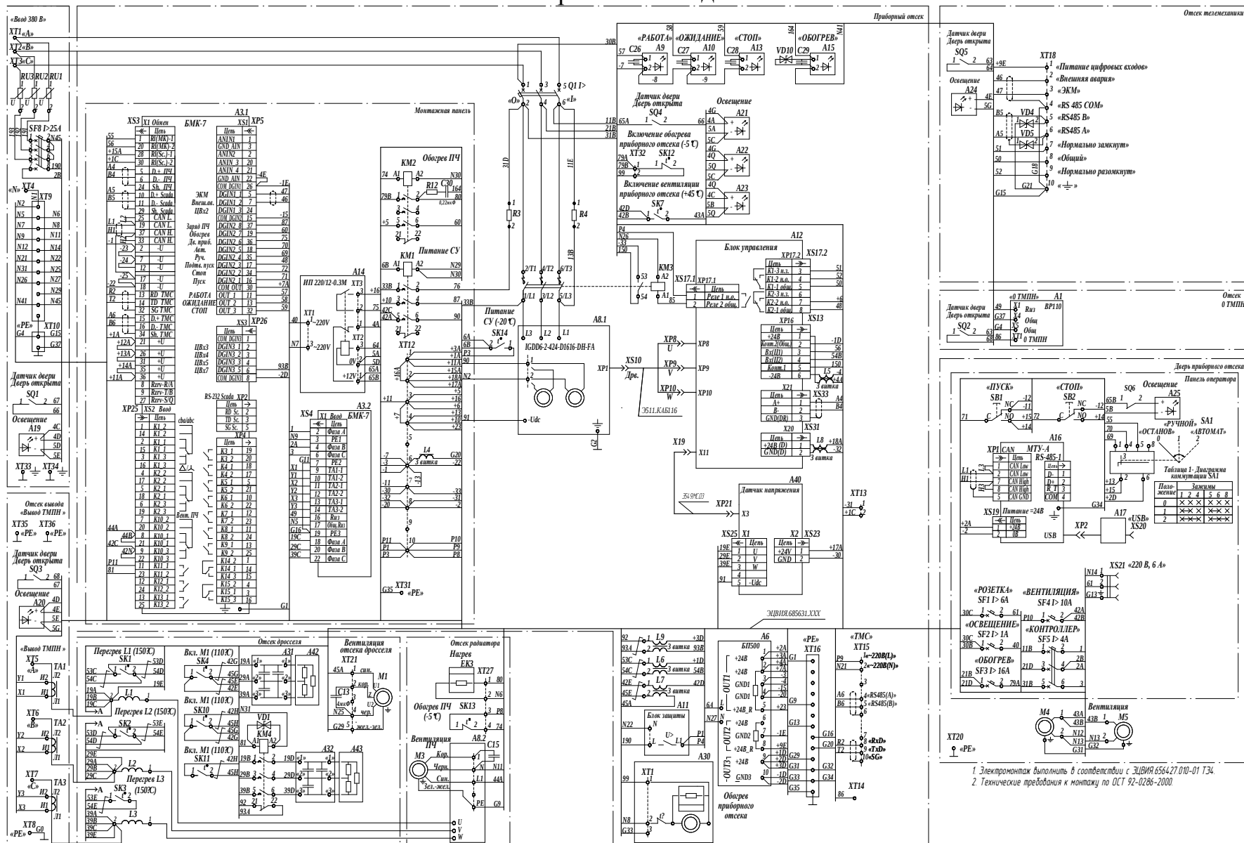
Рисунок Б.1 - СУ ИР3-550
