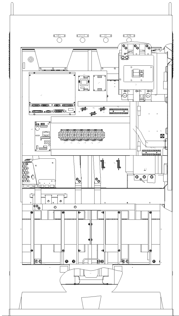
Вид СУ спереди без монтажной панели
